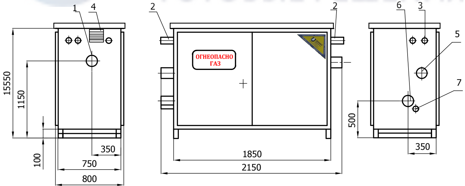
Габаритный чертеж
